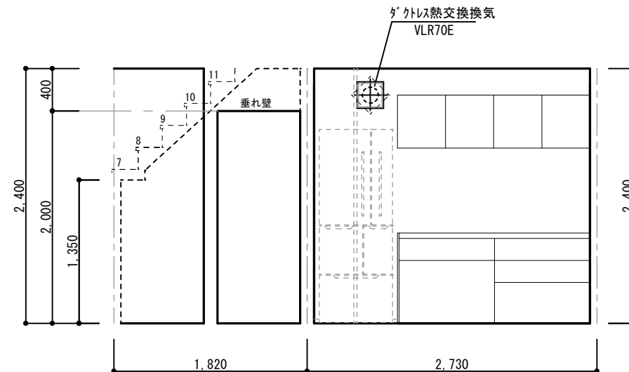
LDK 北面
