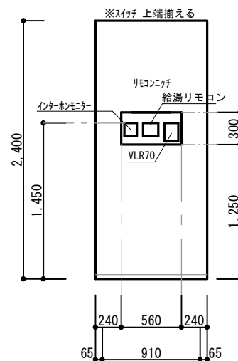
玄関 東面
