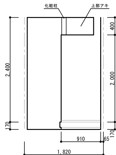
玄関 東面
