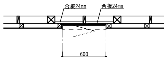
壁掛けTVブラケット用ニッチ 断面図 (1/30)
