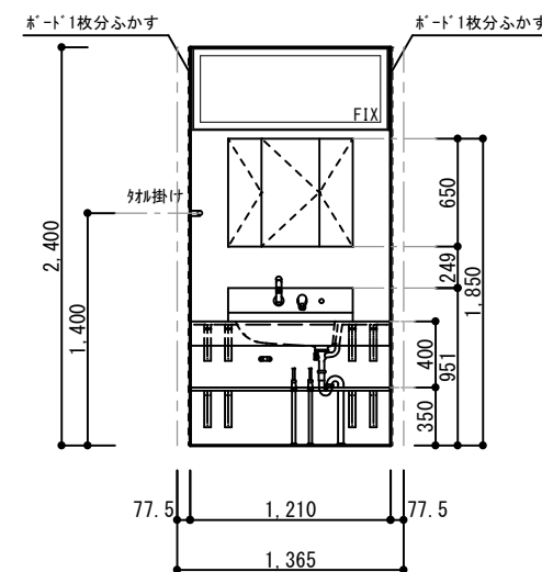
洗面所 西面
