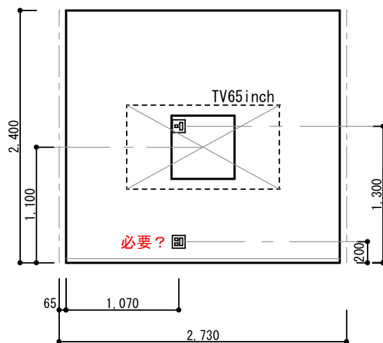
LDK 西面
