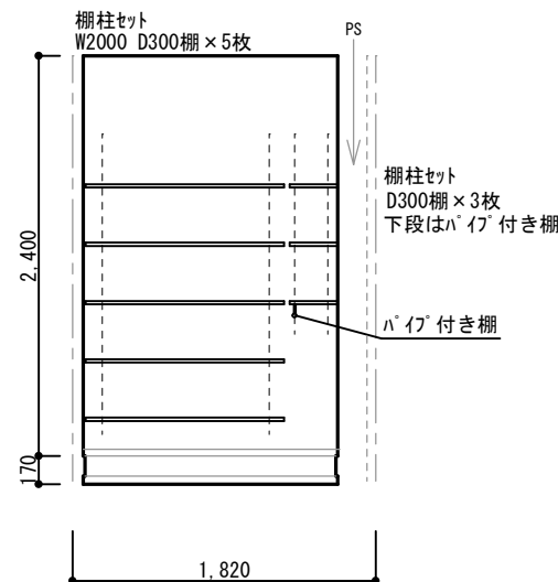
SC 東面
